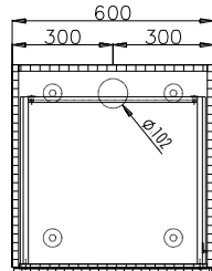
R 63/R 64 Container
