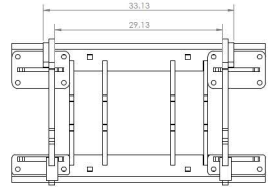
FMT930 JRB 416
