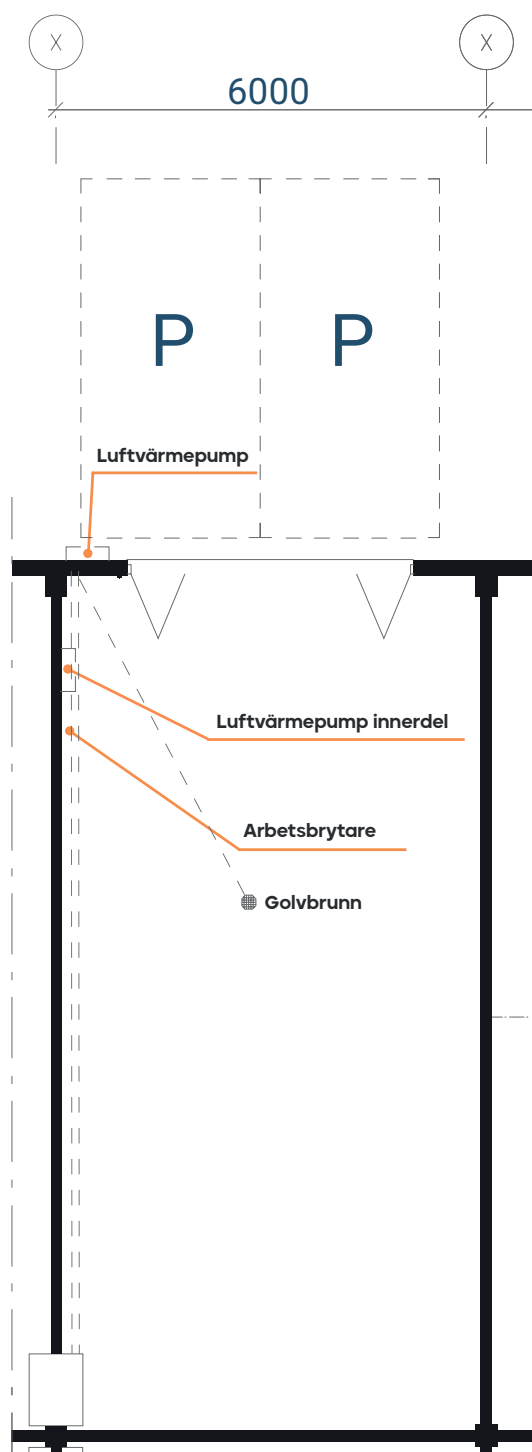
Plan bottenvåning
