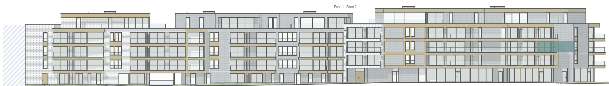
vooraanzicht
