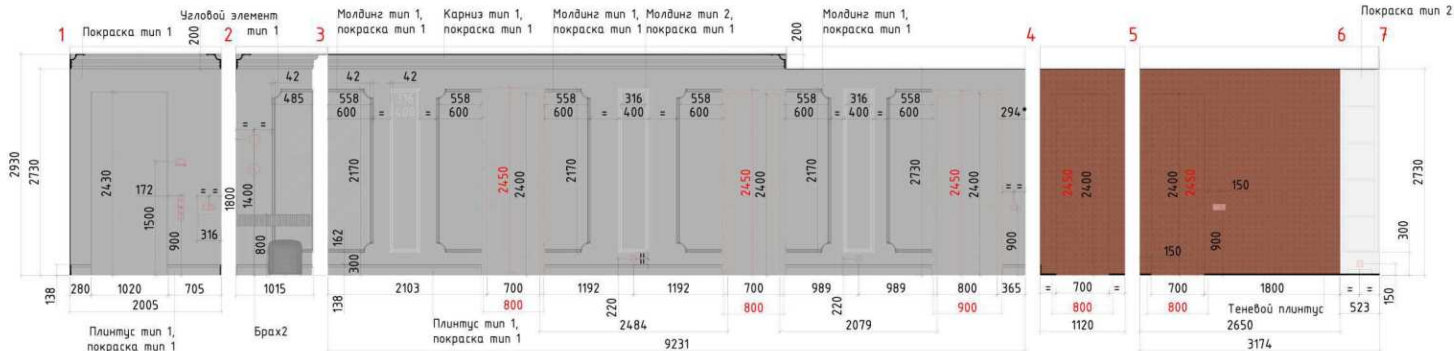
План координации разверток
