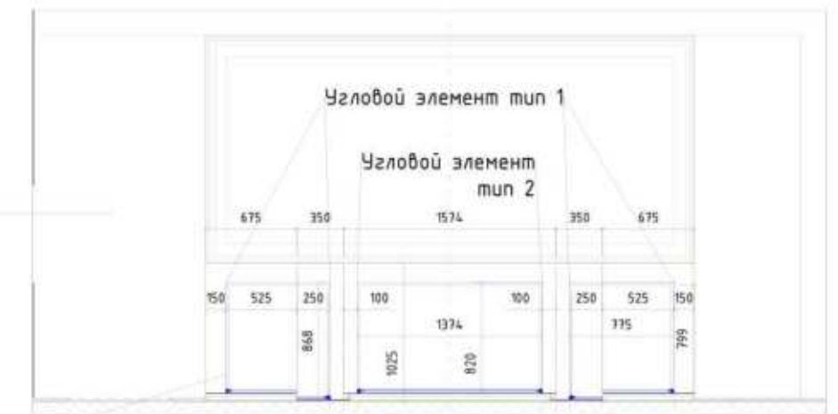
Раскладка потолочных молдингов (пом.13)
