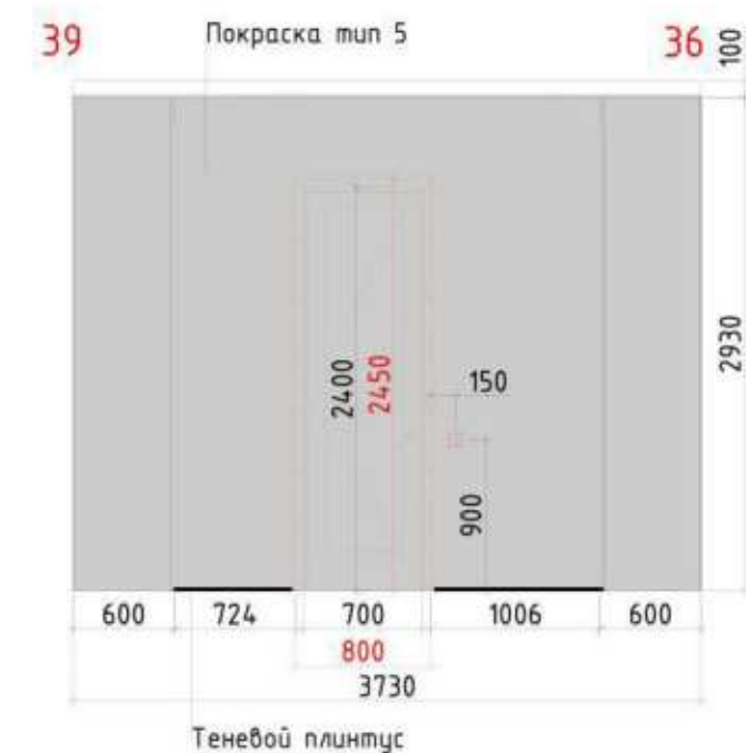
Детская 1 (пом.10)
