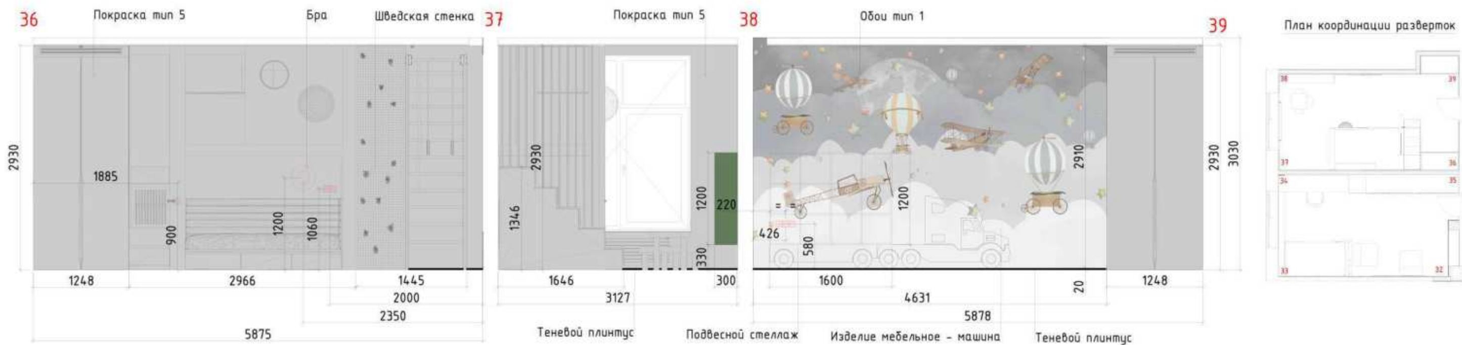
Детская 1 (пом.10)
