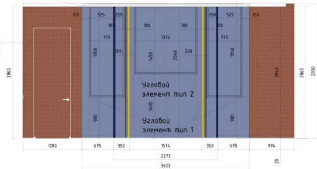
Раскладка настенных молдингов (пом.13)
