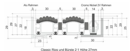
Alumatte Classic - Rips und Bürste 2:1 Höhe 27 mm
