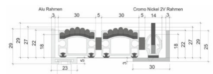
Alumatte Classic - Rips und Bürste 2:1 Höhe 27 mm
