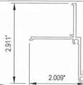
13 SILL CAP DIE # 1060-003 MATERIAL: ALUMINUM ALLOY: 6063-T6 TYPICAL WALL: .072"
