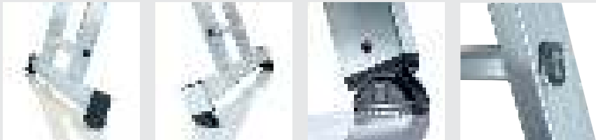
Standard-Traversal nivello® Traverse nivello® Leiterschuhe 4-fach gebördelte Sprossen- / Holmverbindung
