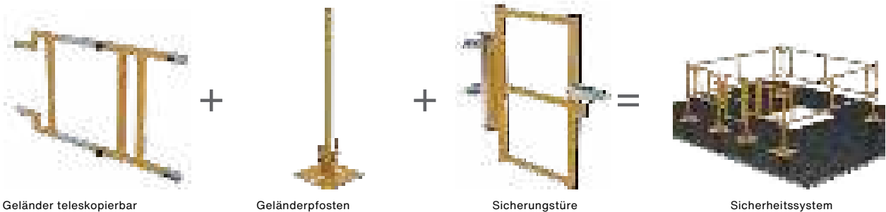
Geländer teleskopierbar
