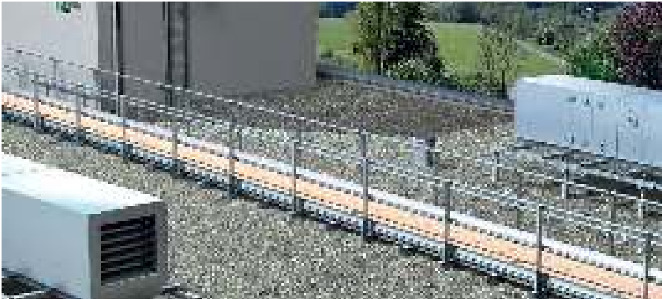
Die Auflast durch den Plattenbelag sorgt für die Standsicherheit des Systems
