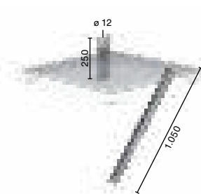
Abb. Bestell-Nr. 60954 (Flanschplatte und Strebe für Ziegelmauerwerk)
