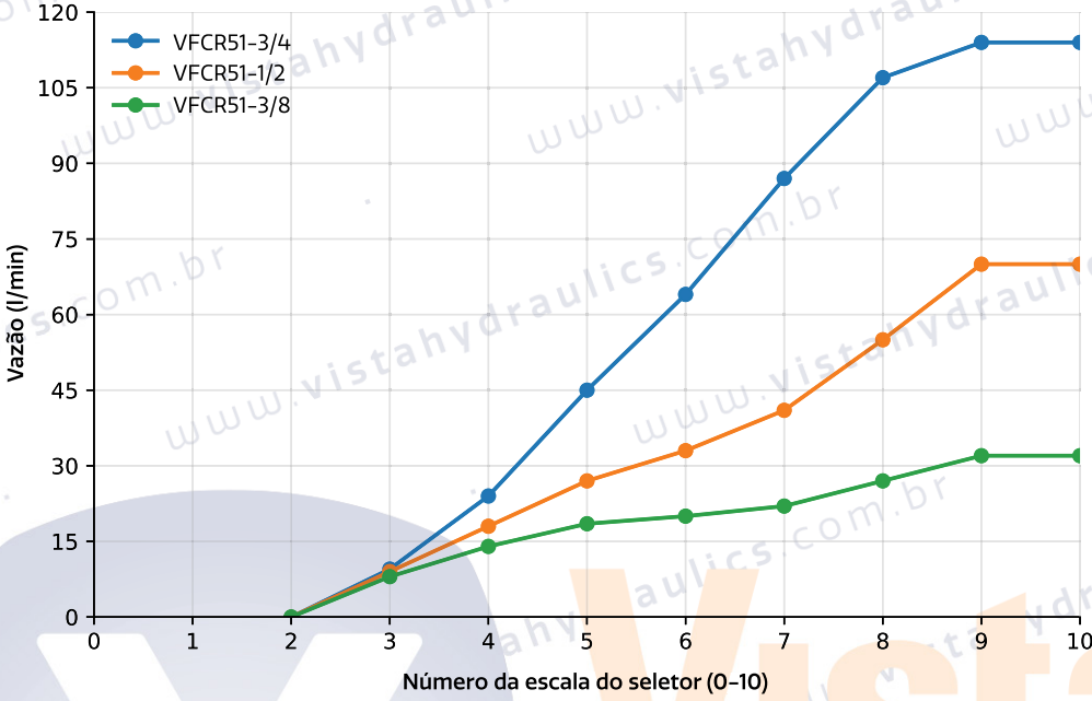
Vazão controlada x posição do seletor – Série VFCR
