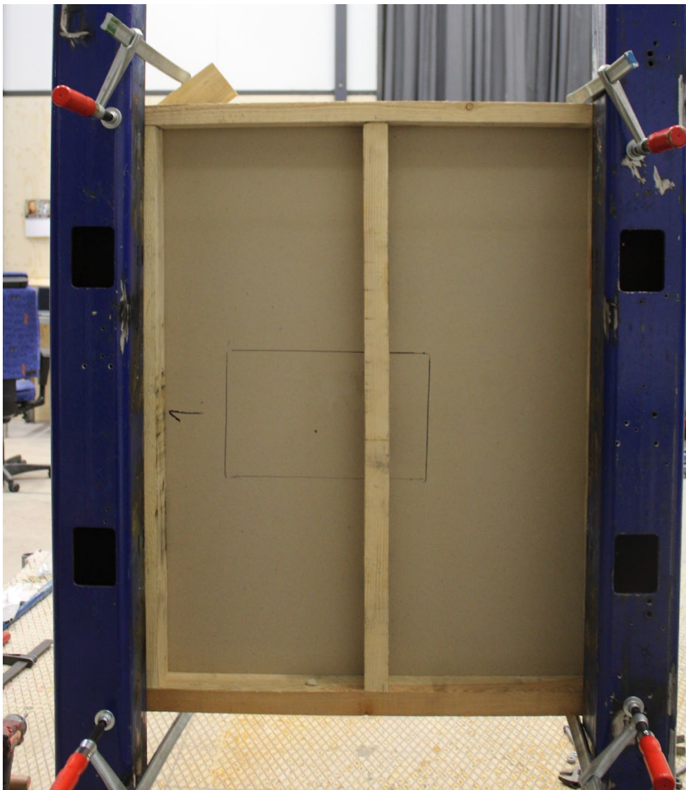
Figur 4 - Provuppställning, Baksida
