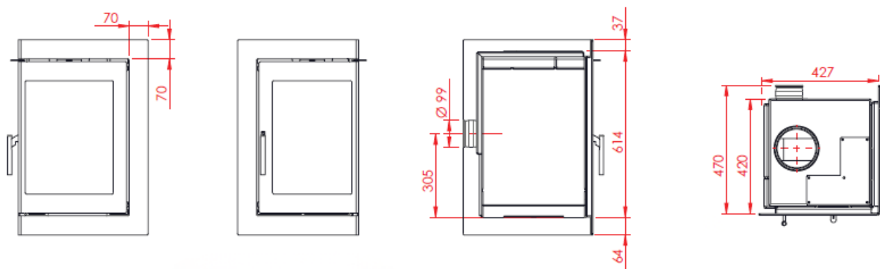
470 højformat med vinkellåge, frisk luft side
