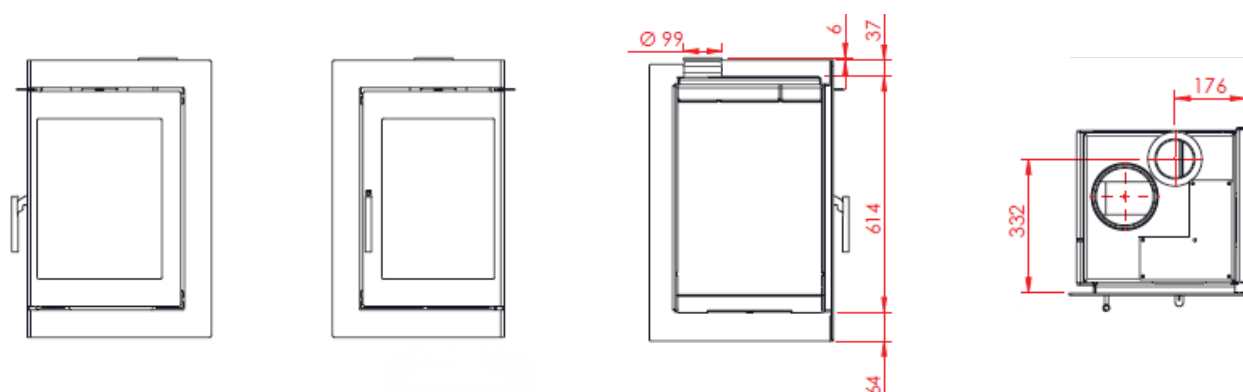
470 højformat med vinkellåge, frisk luft top
