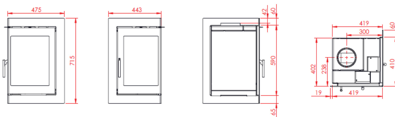
470 højformat med vinkellåge
