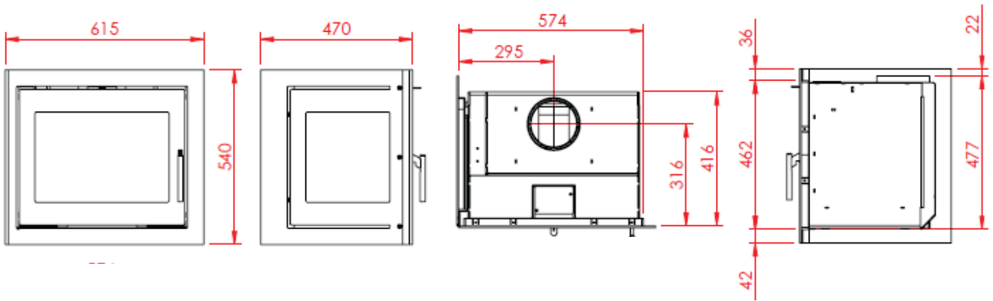
470 fast glas 1 side, frisk luft bag
