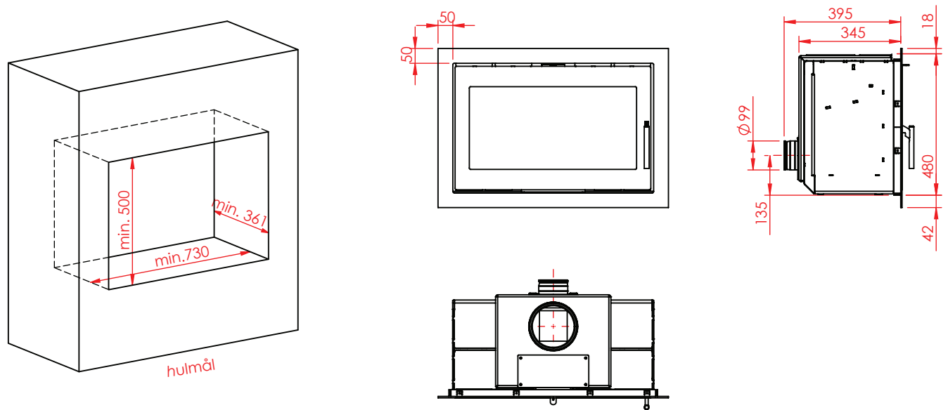
Jupiter 470 XL IR, friskluft bag
