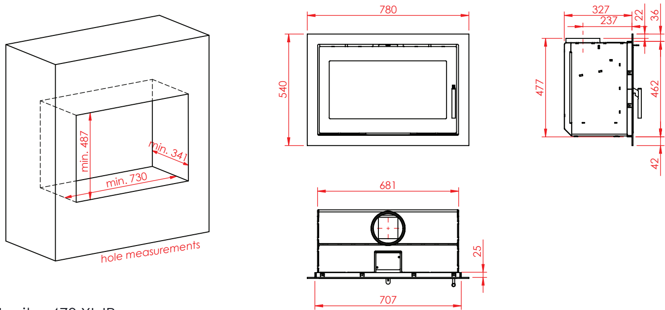
Jupiter 470 XL IR
