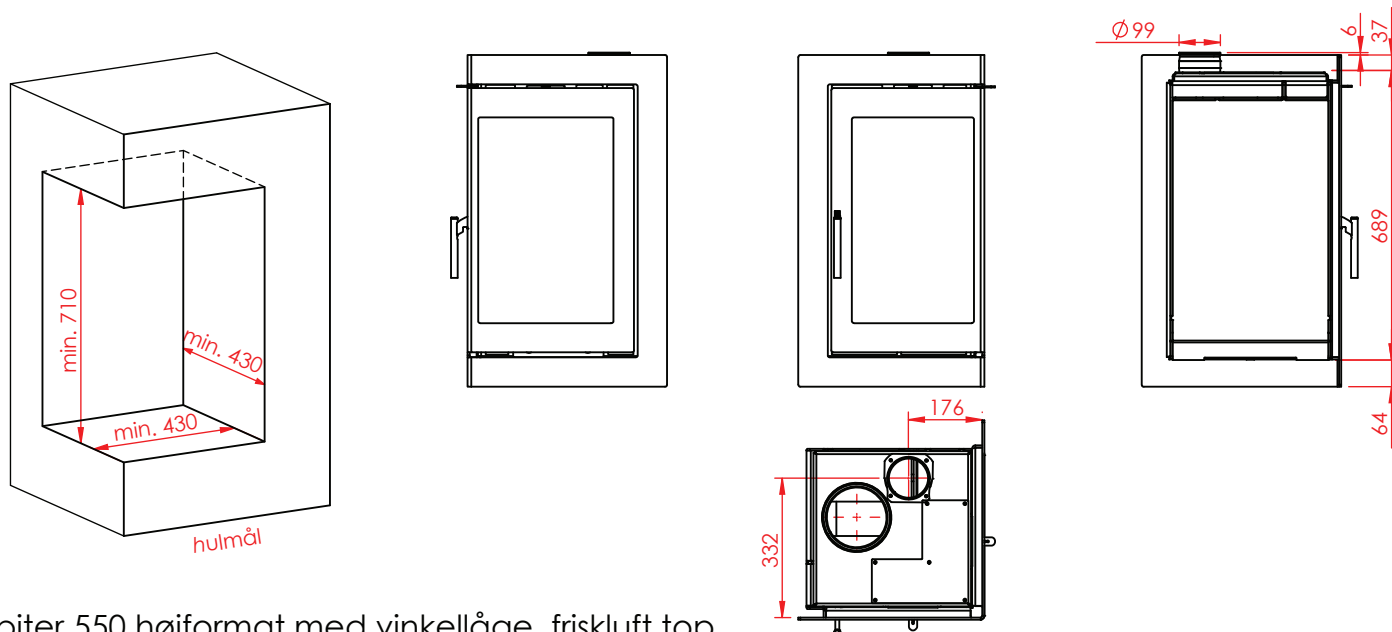
Jupiter 550 højformat med vinkellåge, friskluft side
