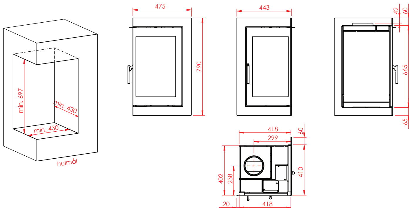
Jupiter 550 højformat med vinkellåge
