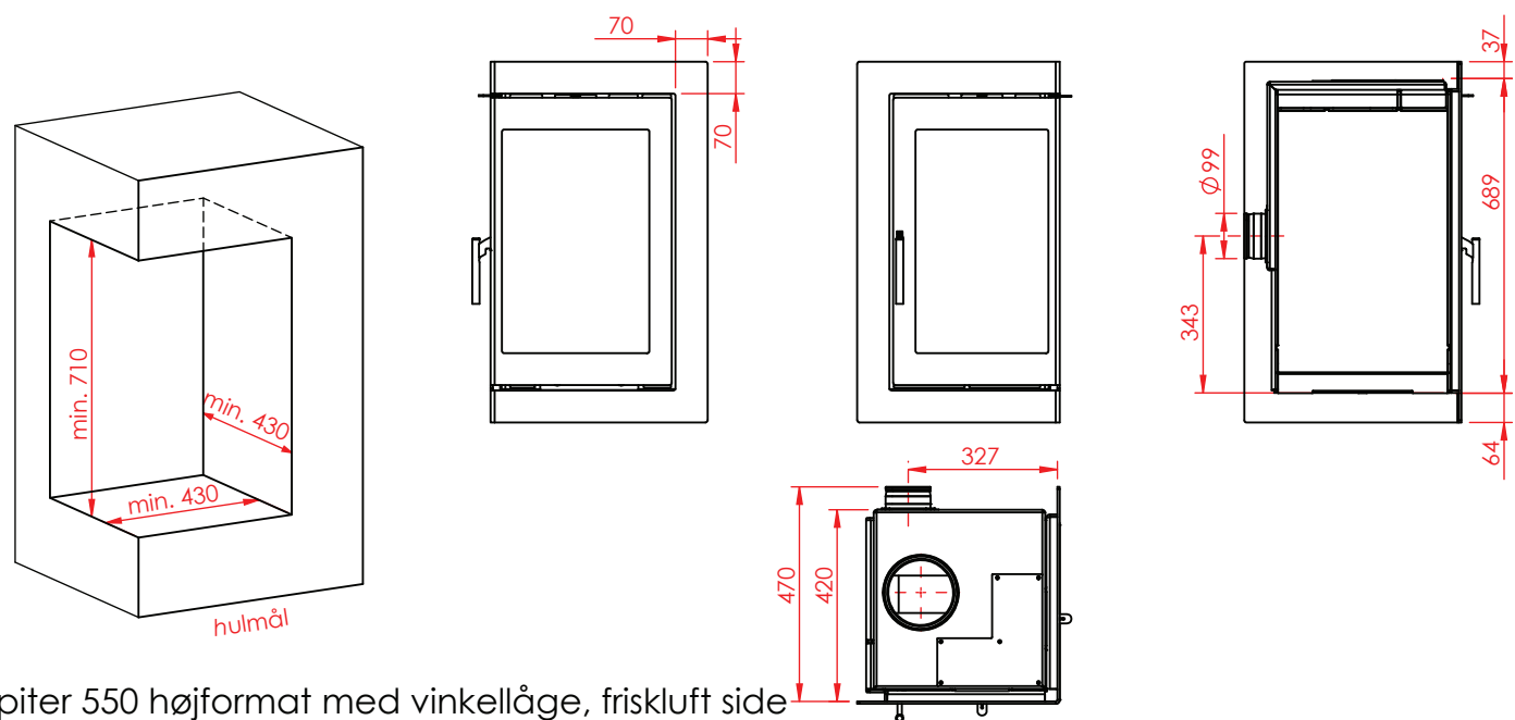
Jupiter 550 højformat med vinkellåge
