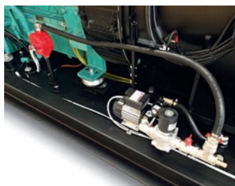
Dispositivo di rabbocco automatico serbatoio Automatic refuelling device Dispositif de remplissage automatique du réservoir
