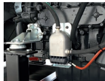
Scaldiglia acqua Water heater Préchauffage de l'eau
