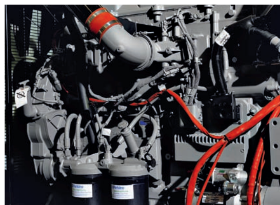
Dettaglio del motore e del fissaggio cavi Detail of the engine and harness Détail du moteur et des câbles
