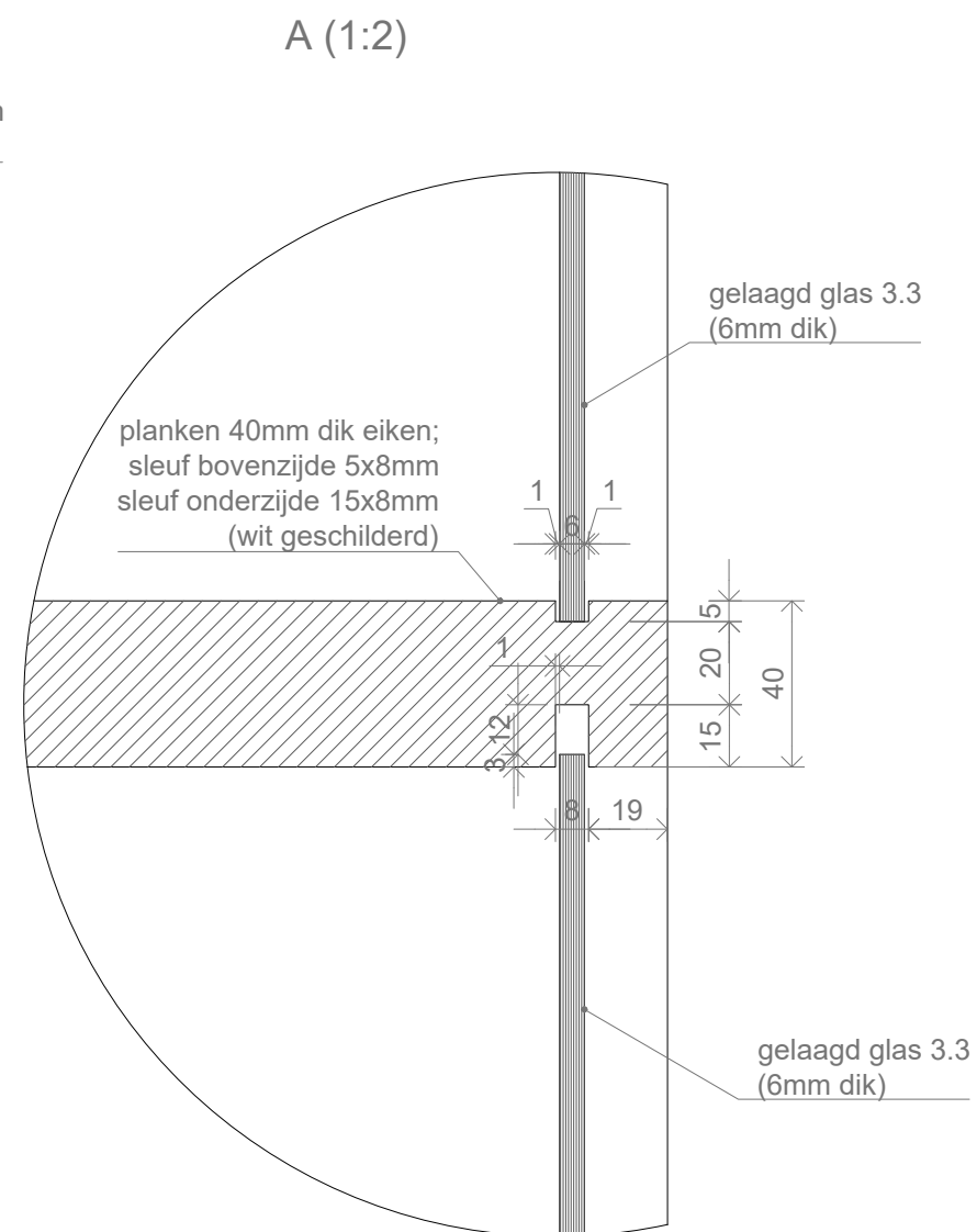
DETAIL: A
