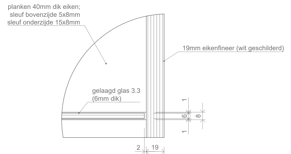
DETAIL: B
