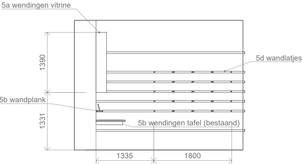
RECHTER ZIJAAANZICHT
