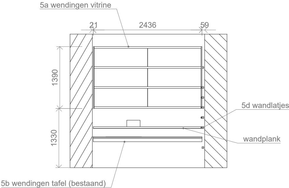
DOORSNEDE A
