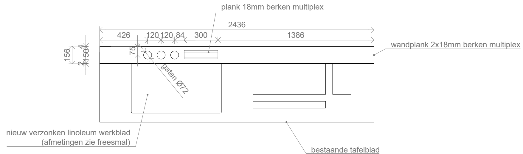
BOVENAANZICHT
