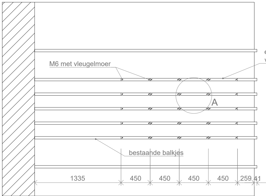
DOORSNEDE B
