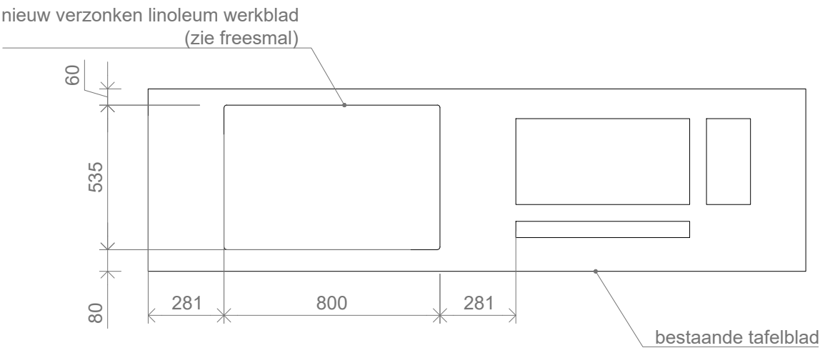
BOVENAANZICHT
