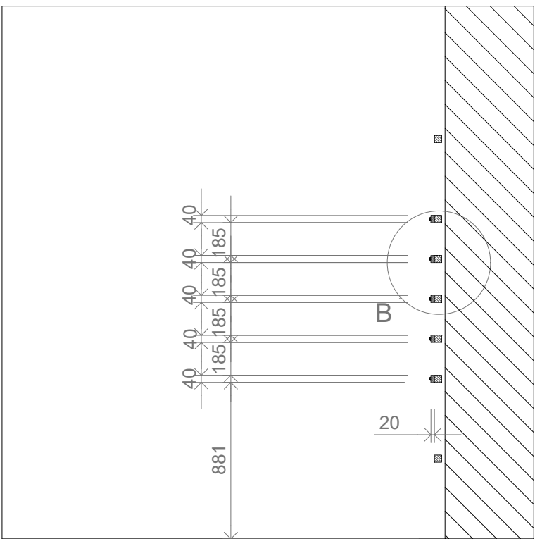
DOORSNEDE C
