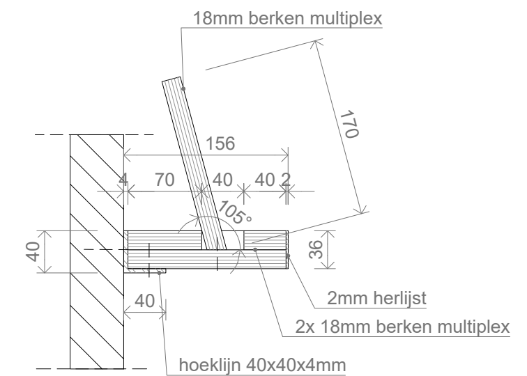
DOORSNEDE A (schaal 1:5)
