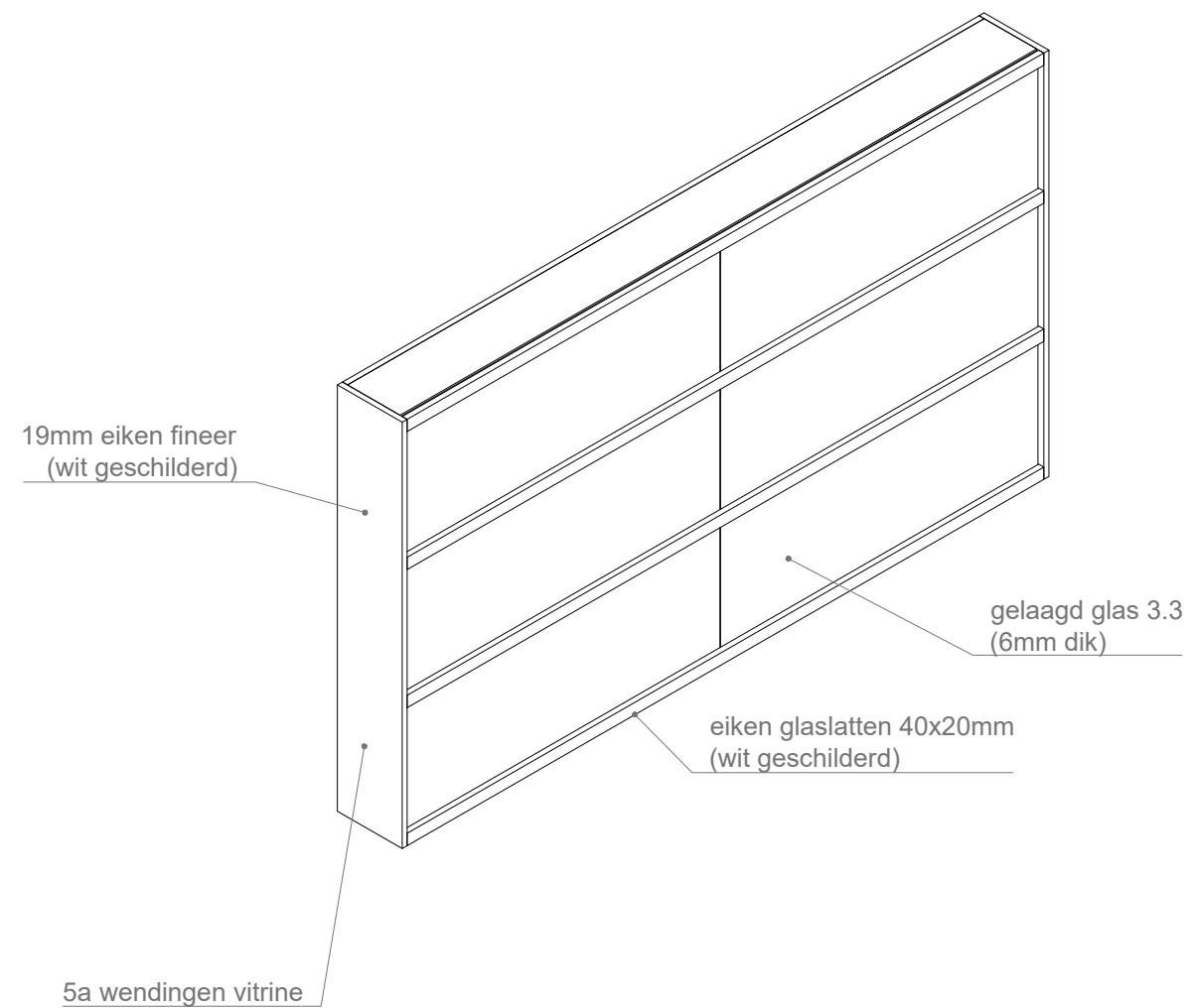
ISOMETRIE VOORZIJDE
