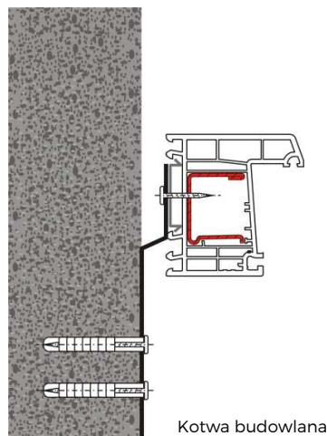
Kotwa budowlana
