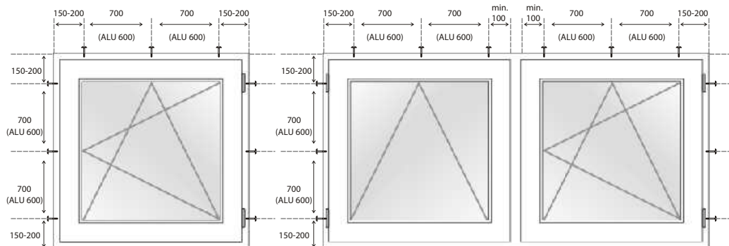
Schemat rozmieszczenia dybli do ram PCV (ALU)
