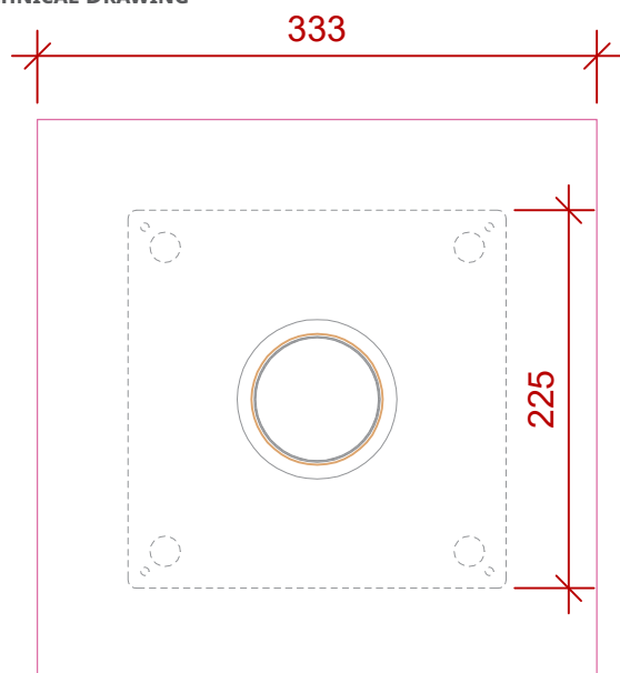
Plan A-A 1:5
