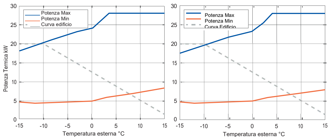
fig. 7: Curve prestazionali della EU20L con deltaT 5K e 85% di umidità (sinistra: temperatura mandata 35 °C / destra: temperatura mandata 55 °C) caratteristica prestazionale secondo EN 14825.
