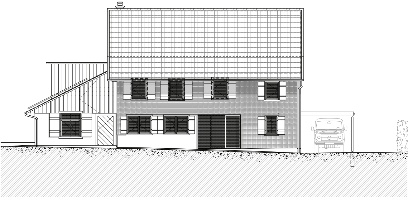
FASSADE SÜD
