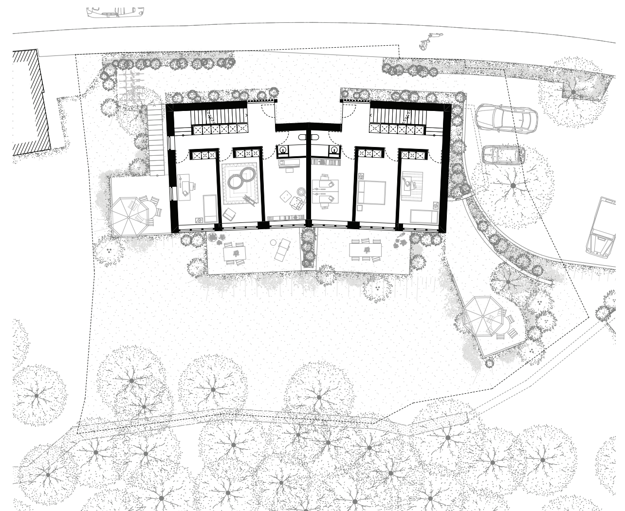
GRUNDRISS EG
