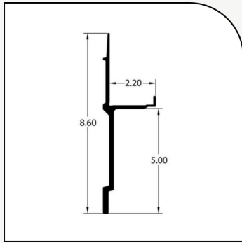
GDP60307101 BORDA INFERIOR GD 623.50
