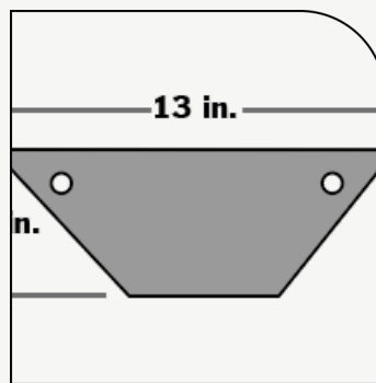
GDP43960005 OREJETA DE APOYO TRIÁNGULO DE APOYO 13 X 4-1/2 X 3/8"
