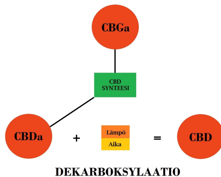
Kuvio 2. Dekarboksylaatio
