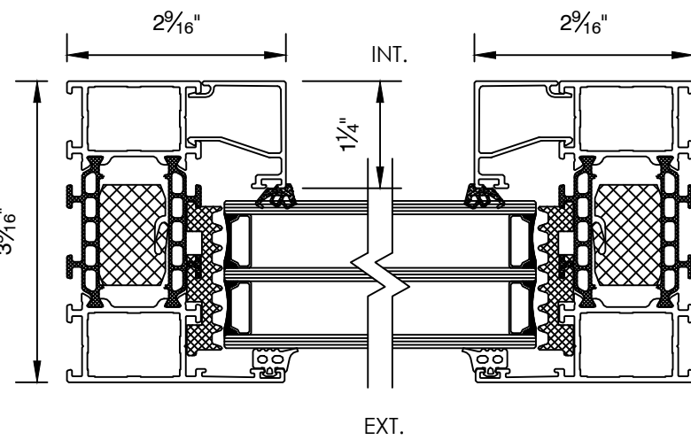
1 JAMB DETAIL SCALE: 6" = 1'-0"
