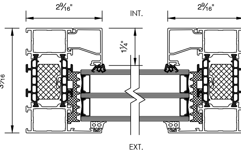
5 JAMB DETAIL SCALE: 6" = 1'-0"
