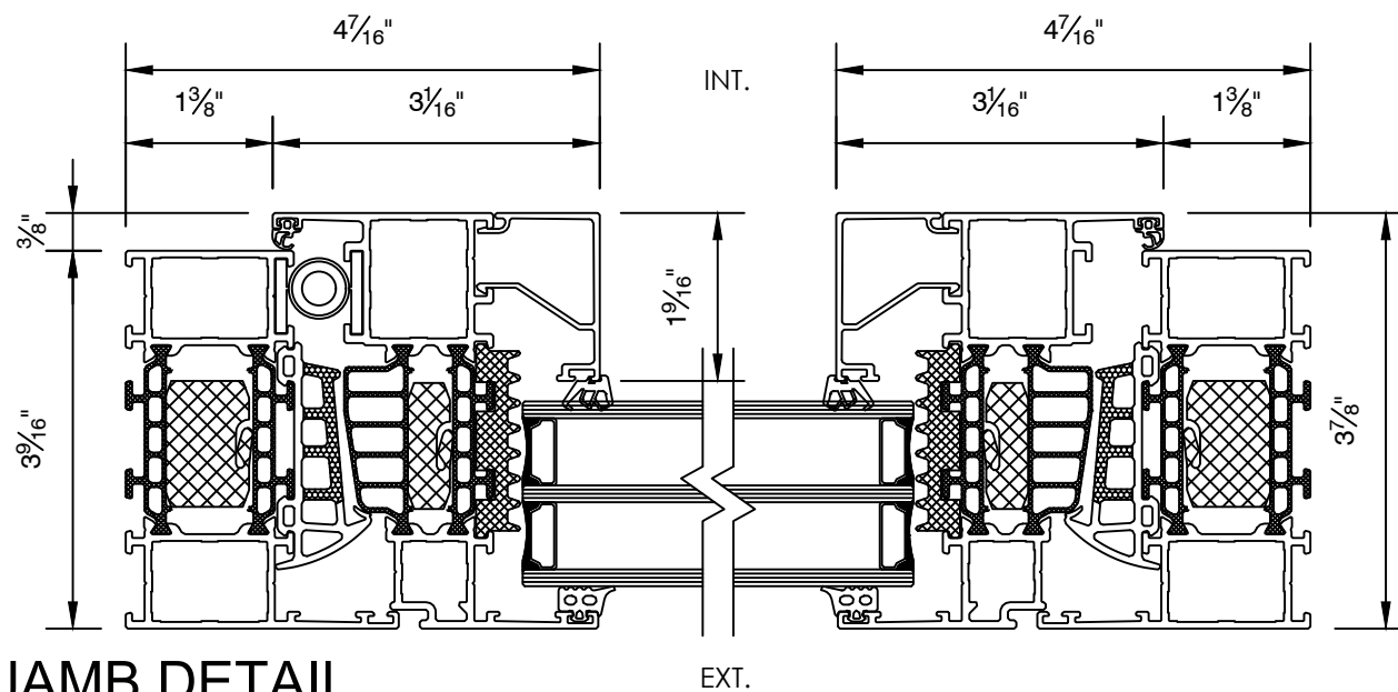
7 JAMB DETAIL SCALE: 6" = 1'-0"
