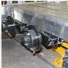
All-aluminum sub-frame
