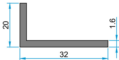
Angle 32x20x1.6
