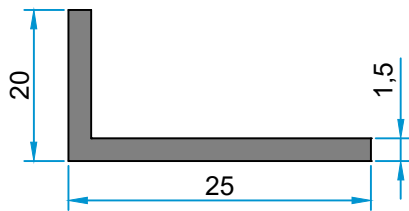
Angle 25x20x1.5mm
