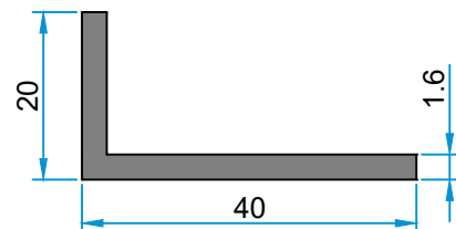
Angle 40x20x1.6
