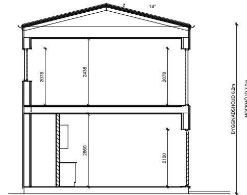
SEKTION B-B
