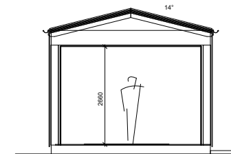
SEKTION C-C
