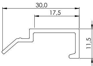
24170 End profile 17,5
