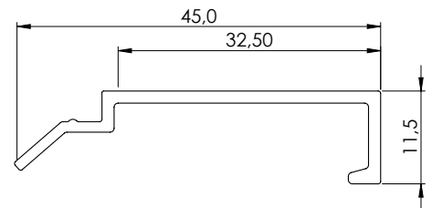
24170-Y End profile 32,5
