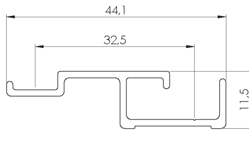
22925 Middle profile 32,5
