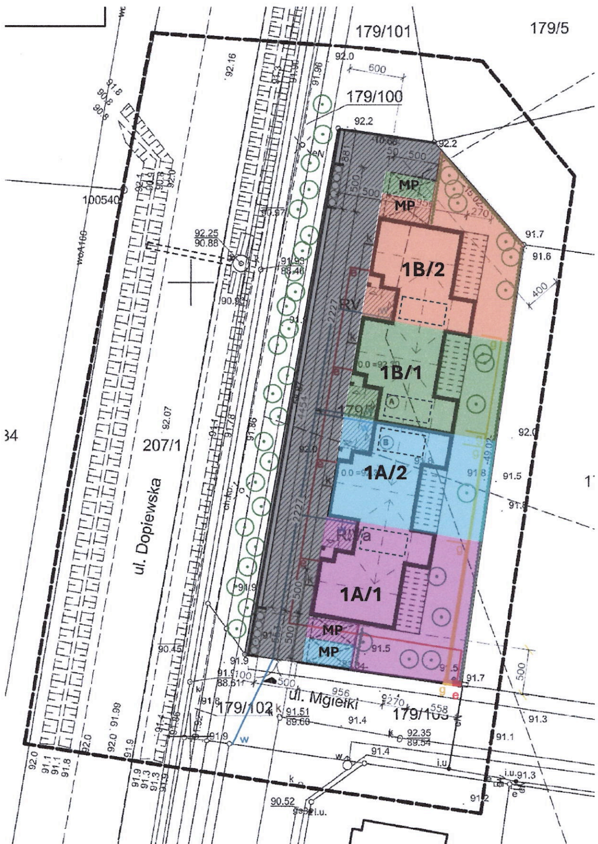
DZIAŁKA NR 179/7 – POWIERZCHNIA 1294 m 2
