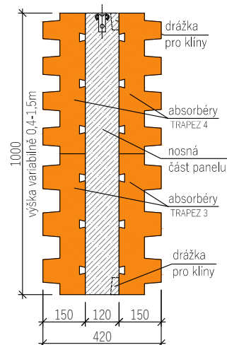
ŘEZ A OBOUSTRANNÝ ABSORBÉR
