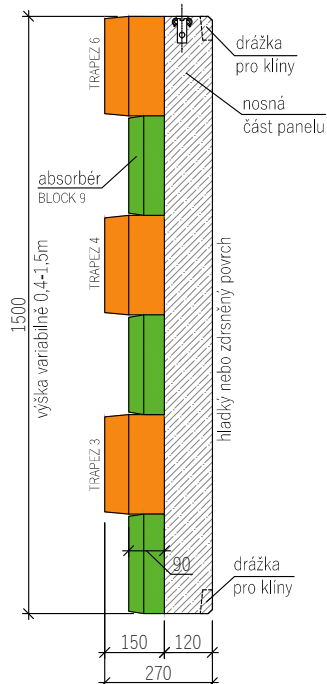
ŘEZ A JEDNOSTRANNÝ ABSORBÉR
