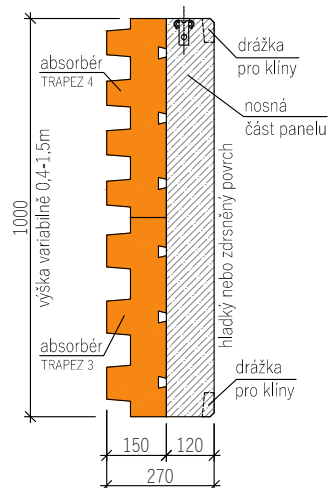
ŘEZ A JEDNOSTRANNÝ ABSORBÉR
