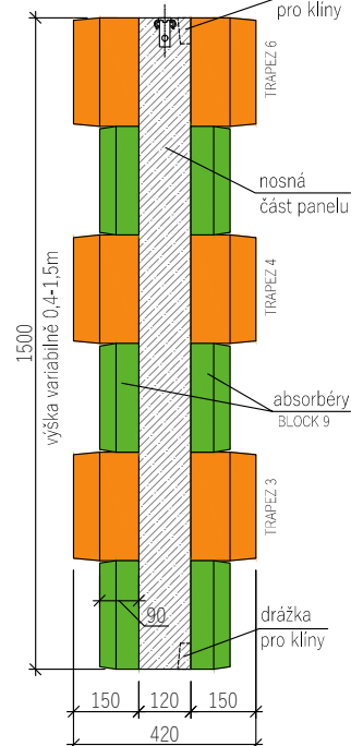
ŘEZ A OBOUSTRANNÝ ABSORBÉR
