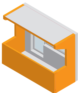
ROVNÁ SE STĚNOU VYBRANOU s betonovým zábradlím
