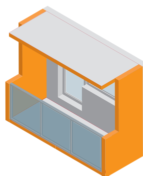
ROVNÁ SE STĚNOU ZŮŽENOU s hliníkovým zábradlím
