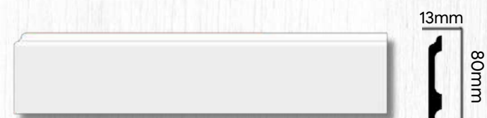
CPU 8013 L: 2400mm W: 80mm
