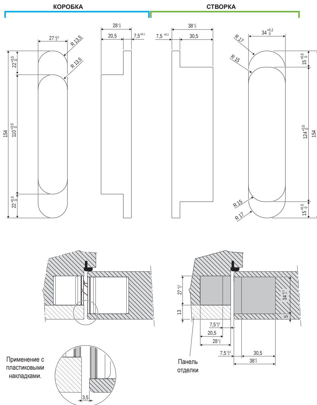
ЧЕРТЕЖ ФРЕЗЕРОВКИ
