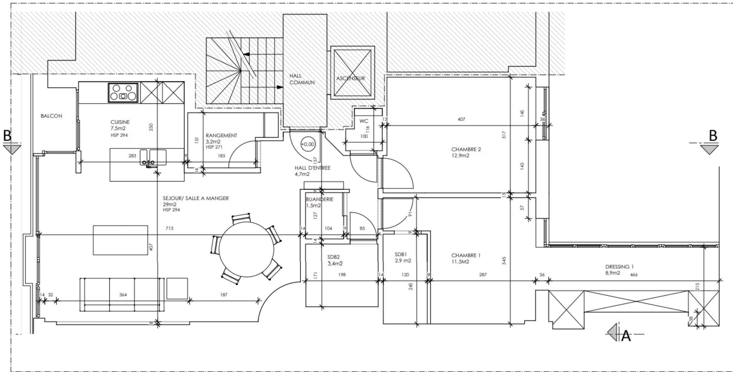
PLAN - APPARTEMENT R+1
