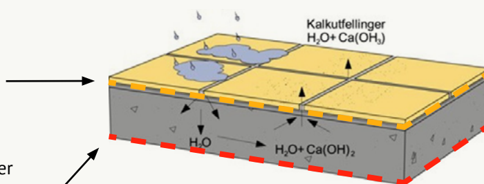
Figur 1: Prinsipper for membranplassering. Figuren viser hvordan fukt vandrer i konstruksjonen avhengig av membranplasseringen.
