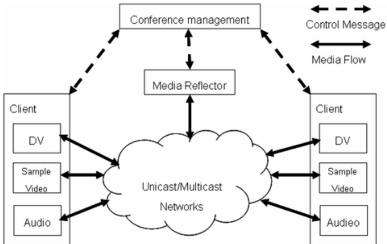
Figura 2 - Arquitetura da vídeo conferência, ref.: DOI:10.1109/IPC.2007.44
