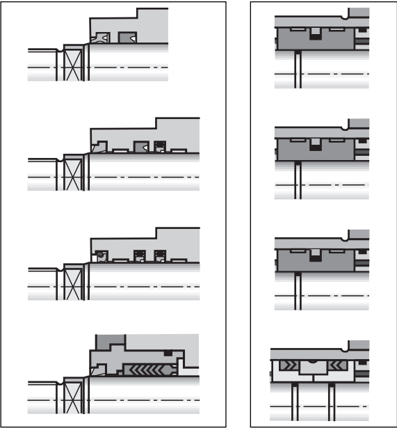
Piston
