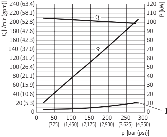
V = 140 cm 3 /rev
