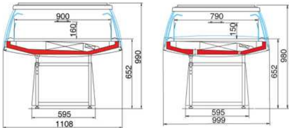
Arrow C Max
