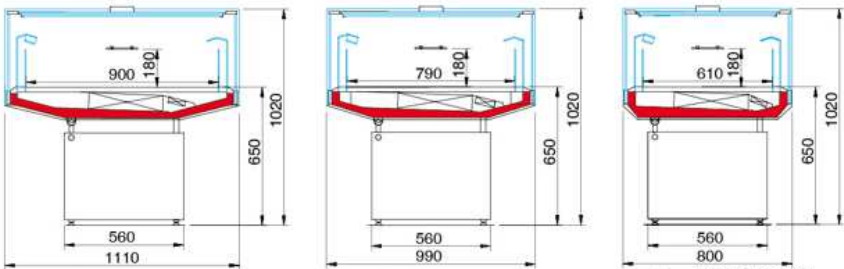
Arrow VD P90 C18 XP
