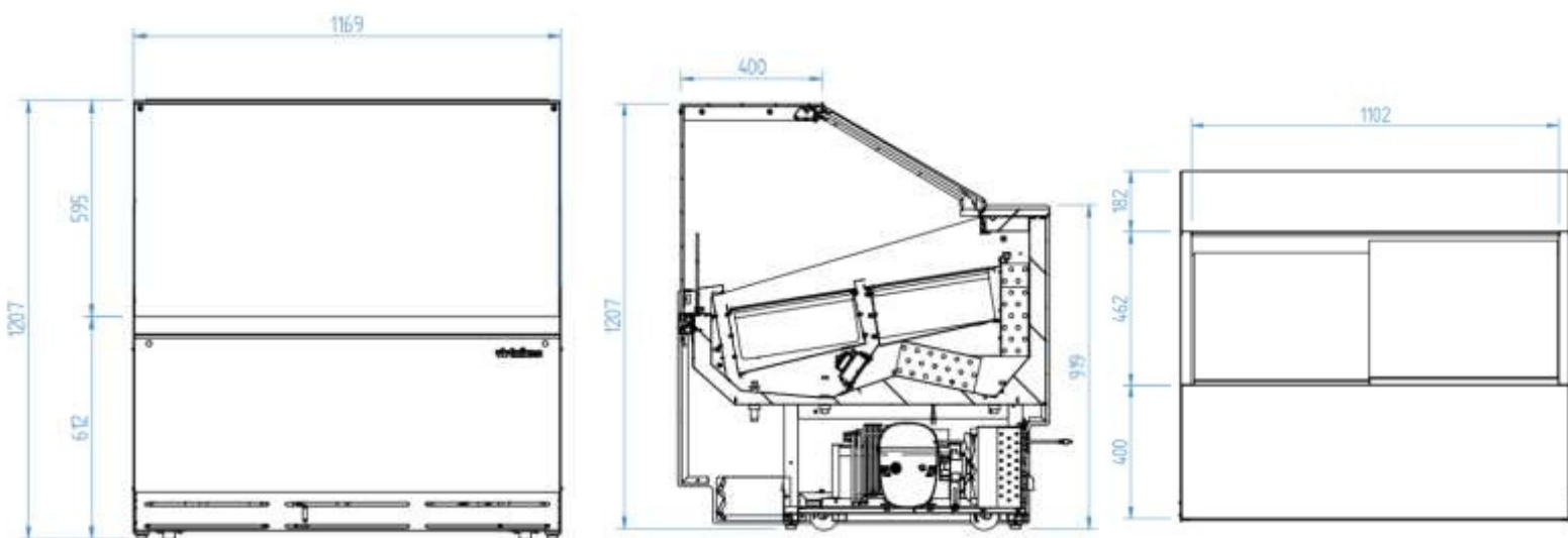
ELEVATION
