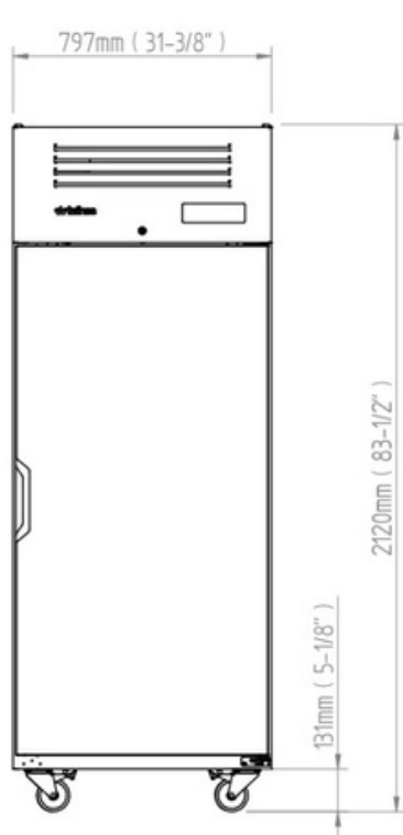
ELEVATION
