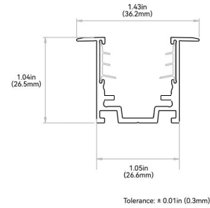
TOP BEND
