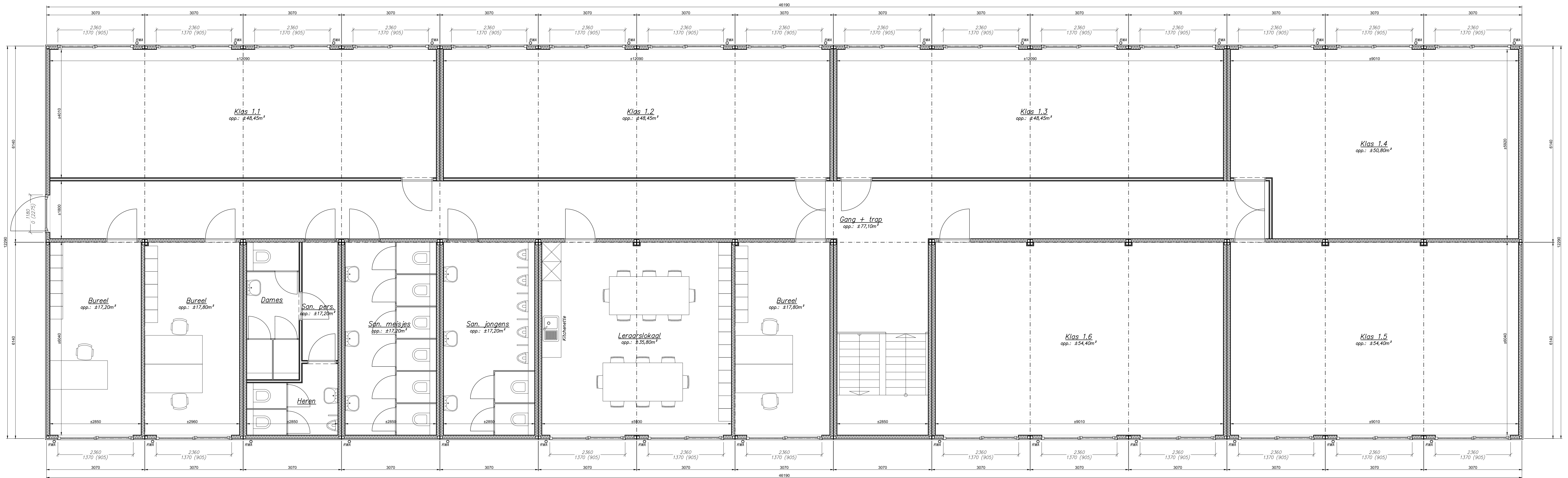
Plan 1e verdieping
