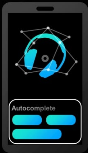
Typeless Input
