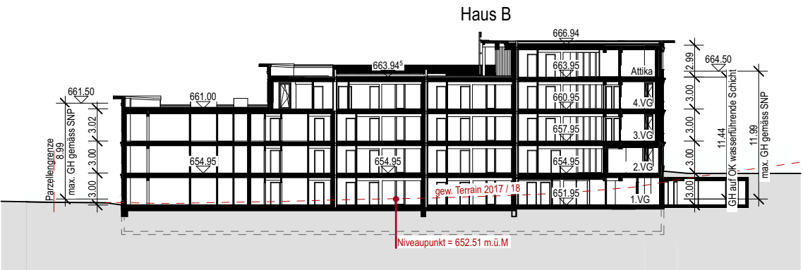
Haus B | Schnitt 3-3
