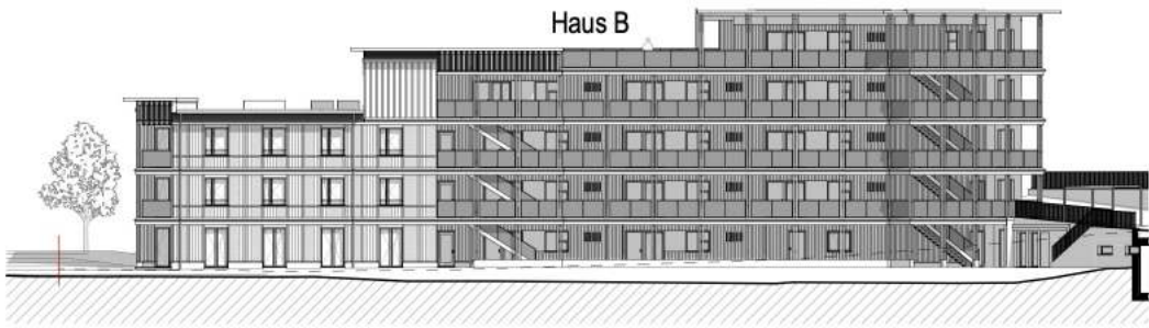
Ansicht Ost
