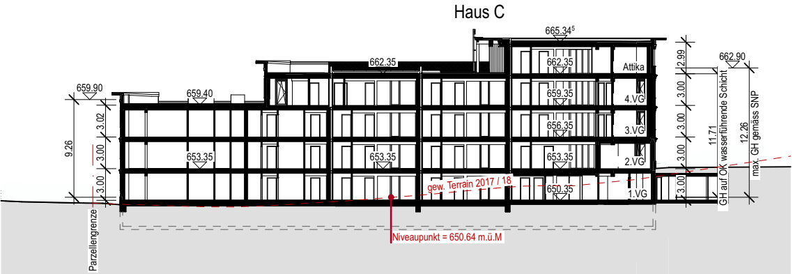
Haus C | Schnitt 4-4
