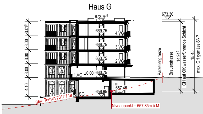
Haus G | Schnitt 1-1
