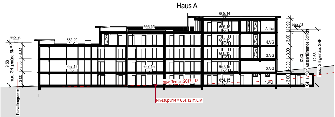
Haus A | Schnitt 2-2
