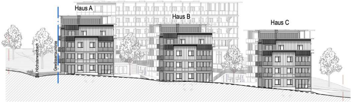
Ansicht Süd
