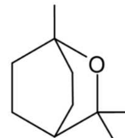
1,8-cinéole
