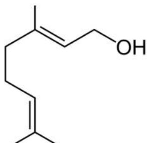
Géraniol
