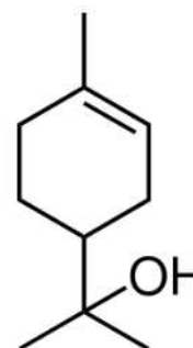
alpha-terpinéol
