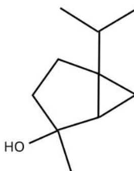
4-Thujanol
