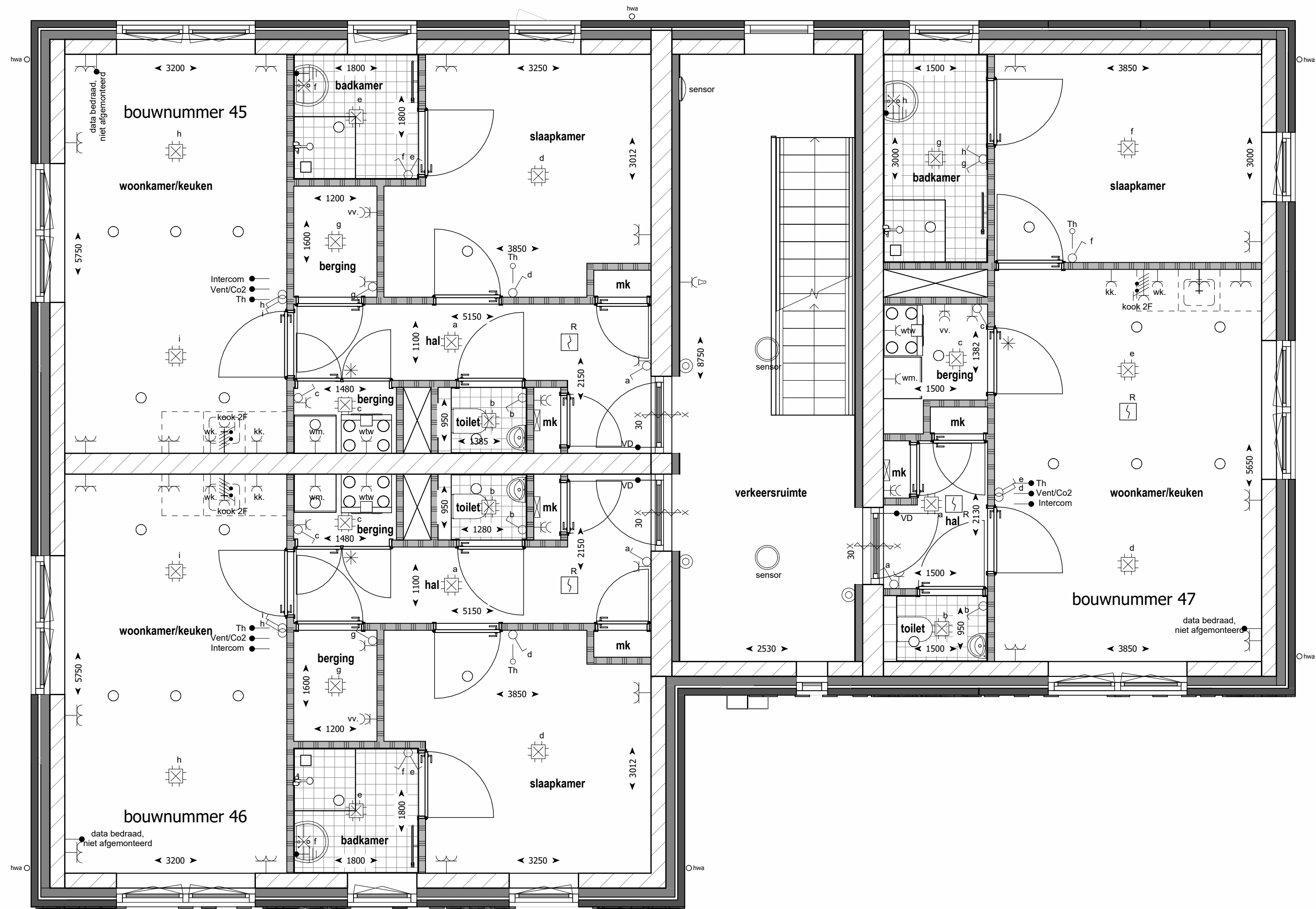
1e verdieping 1 : 50
