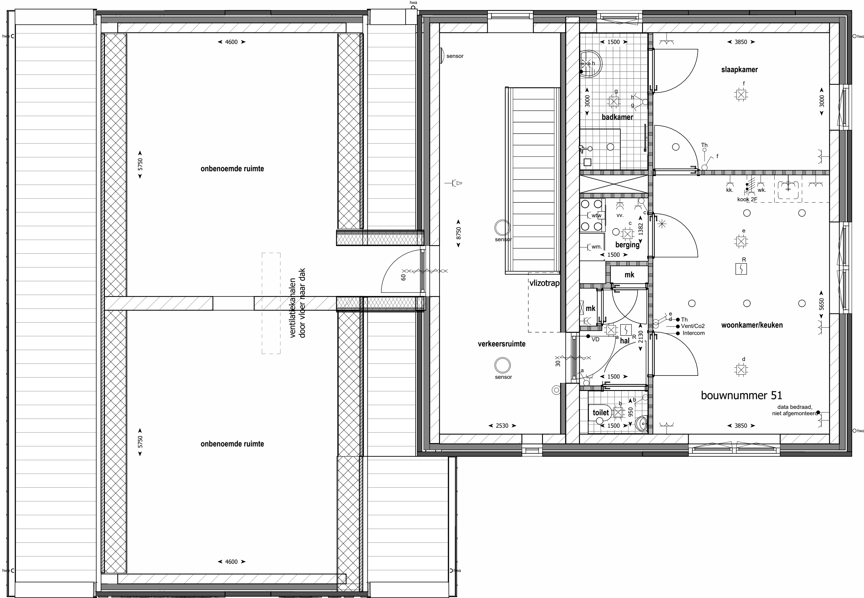
3e verdieping 1 : 50
